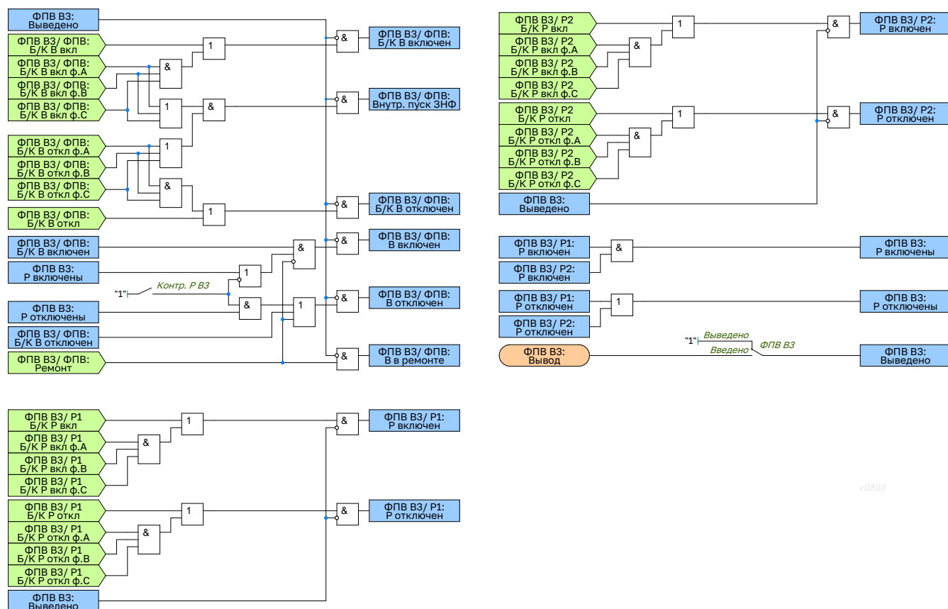
Рисунок 1.59 – Функциональная схема логики ФПВ ВЗ
