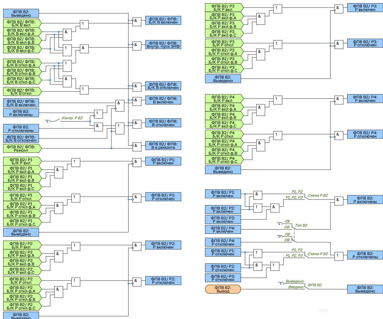
Рисунок 1.58 – Функциональная схема логики ФПВ В2
